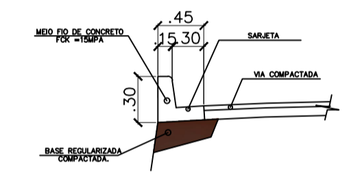
DETALHE SARJETADA sem escala
